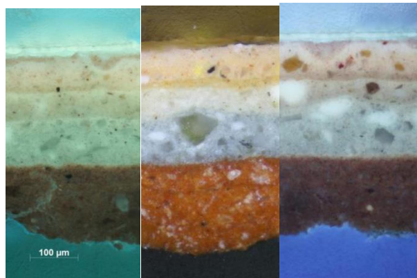
Tisztítópróba (Szent Vendel) A keresztmetszetcsiszolat mikroszkópos felvétele normál, UV és BV megvilágításban jól megkülönböztethetőek a többretegű színes olajalapozás is a festett rétegek felépítése
